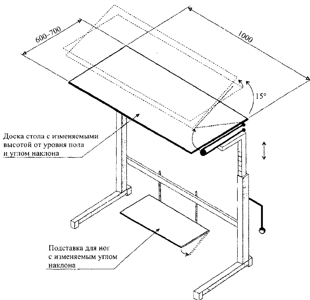
Рисунок В.12. Трансформируемый рабочий стол для инвалида
