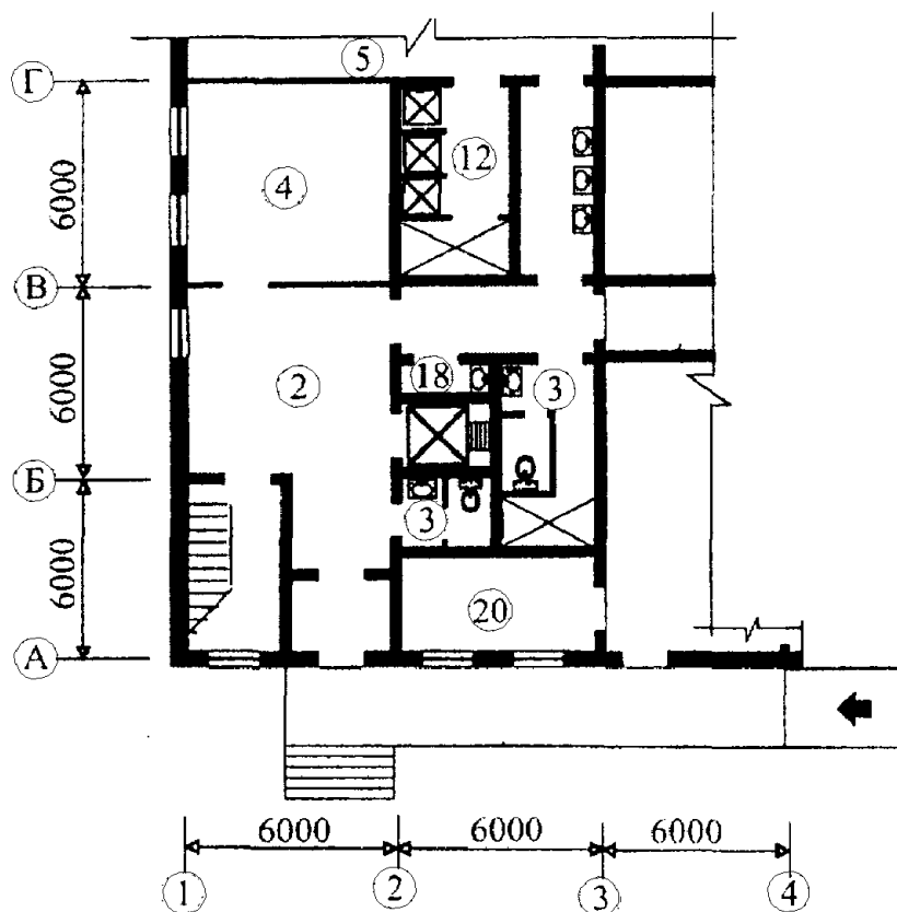
Фрагмент плана на отм. 4.800
