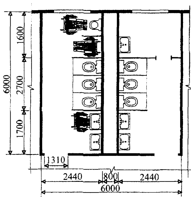
Цеховая уборная с кабиной для инвалидов
