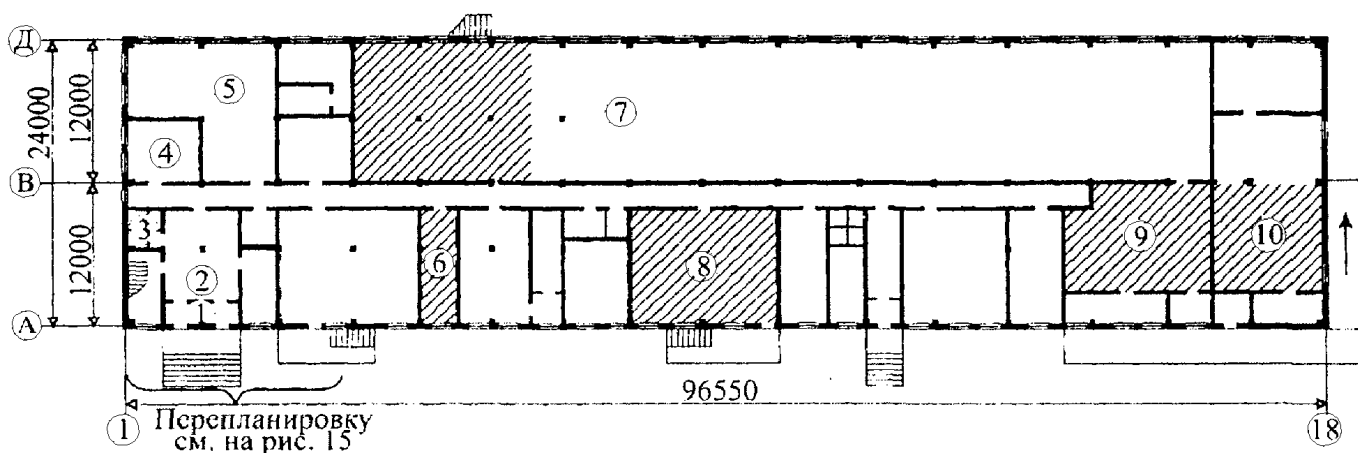
План на отм. 4.800
